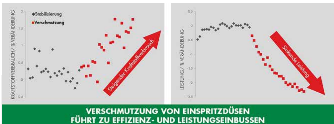
Grafik 1: Die Grafik zeigt die signifikanten Auswirkungen verschmutzter Injektoren auf Kraftstoffverbrauch und Leistung³.
